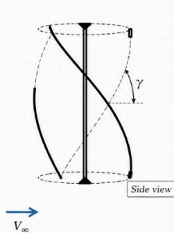
(d) Helical Darrieus
