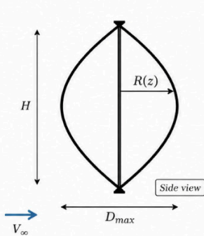
(c) Troposkein Darrieus
